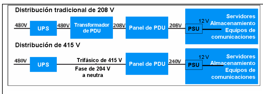
Figura 13. La distribución de energía de 415 V proporciona una alternativa más eficiente para utilizar la energía de 208 V.
